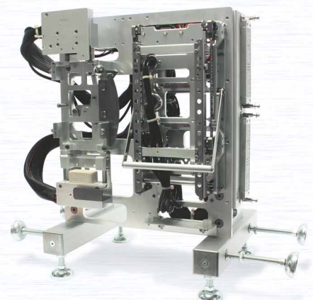
Steuergeräte-Prüfstand zur Temperatur-Zyklusprüfung
